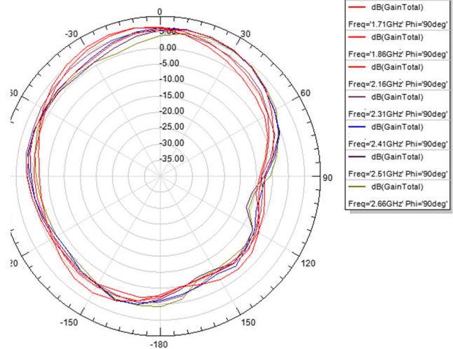
1710MHz, 1860MHz, 2160MHz, 2310MHz, 2410MHz, 2510MHz, 2660MHz Vertical Plane
