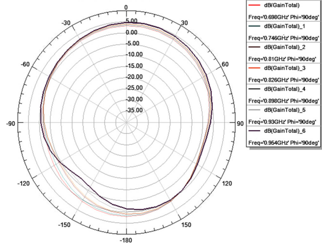
698MHz, 746MHz, 810MHz, 826MHz, 898MHz, 930MHz, 954MHz Vertical Plane
