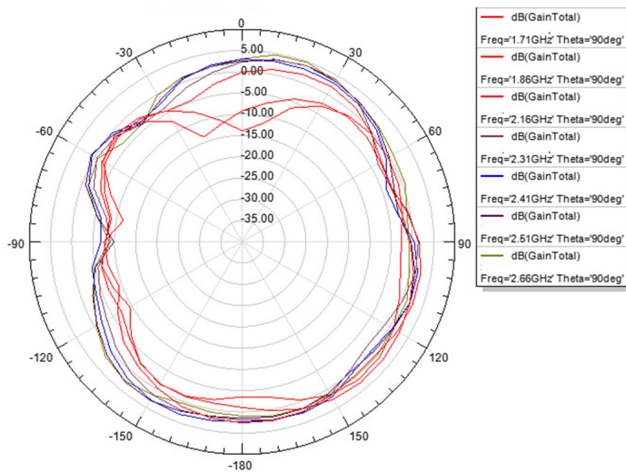
1710MHz, 1860MHz, 2160MHz, 2310MHz, 2410MHz, 2510MHz, 2660MHz Horizontal Plane
