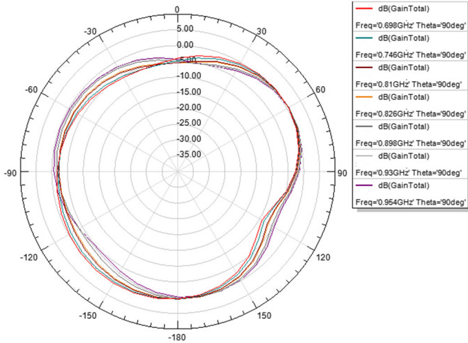
698MHz, 746MHz, 810MHz, 826MHz, 898MHz, 930MHz, 954MHz Horizontal Plane
