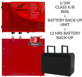
½W ProtectLink™ Kit CS45-727-827-K2
